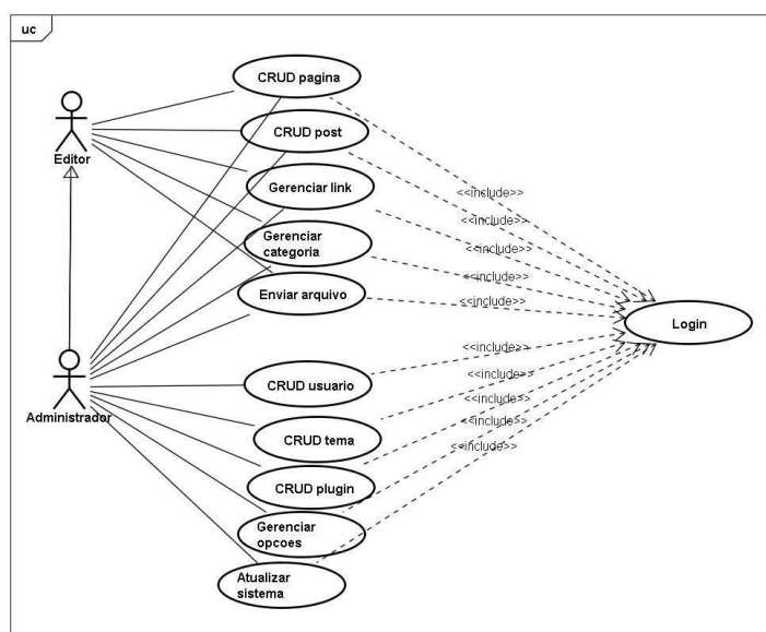
Figura 3: Interação do sistema com o tipo de usuário do site CMDCA.
